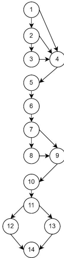
Gambar 7.2 Flow Graph Method buatJadwalKonseling()
